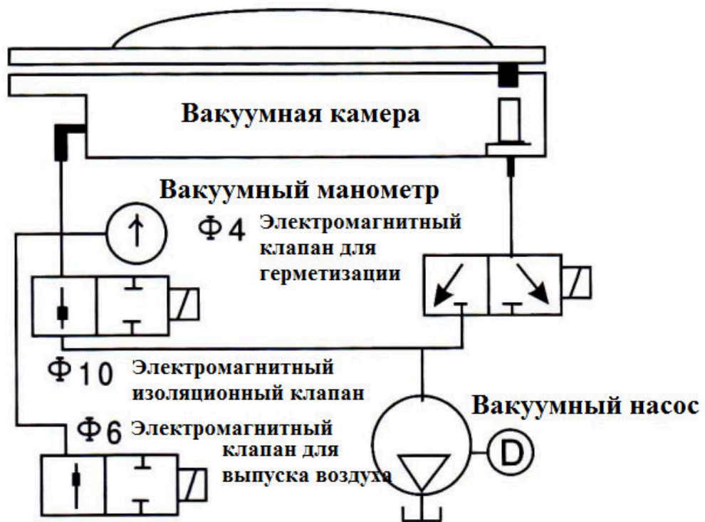
Схема системы откачки воздуха (вакуумной системы)
